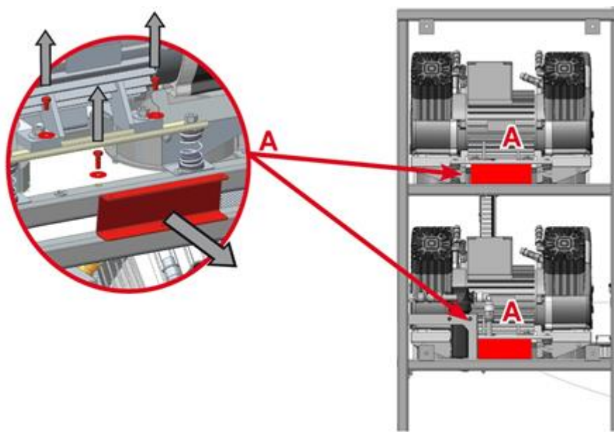
Obr. 6 :Odfixovanie agregátov
