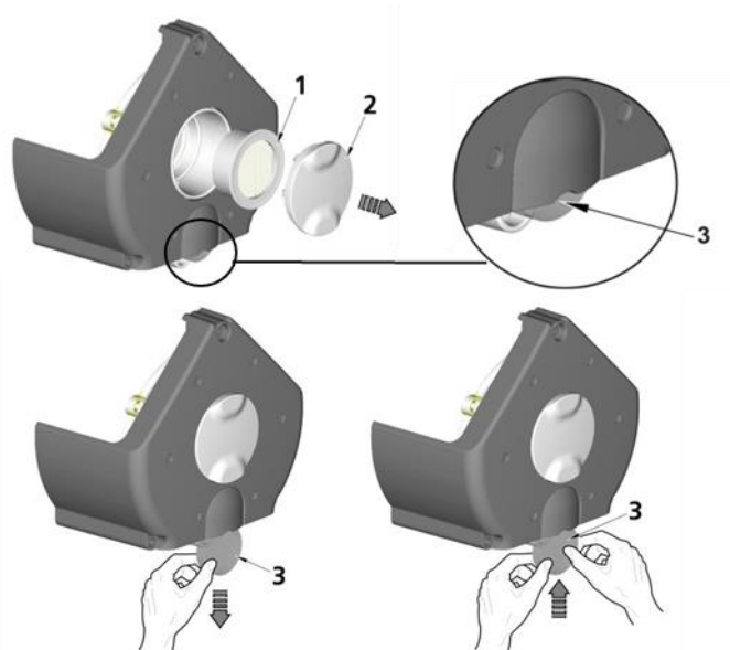
Obr. 24: Výmena vstupného filtra
