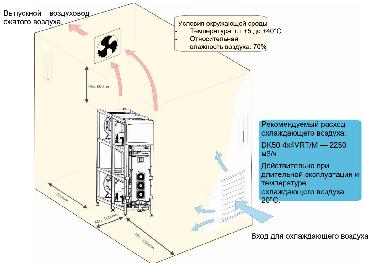
Рис. 4: Установка оборудования
