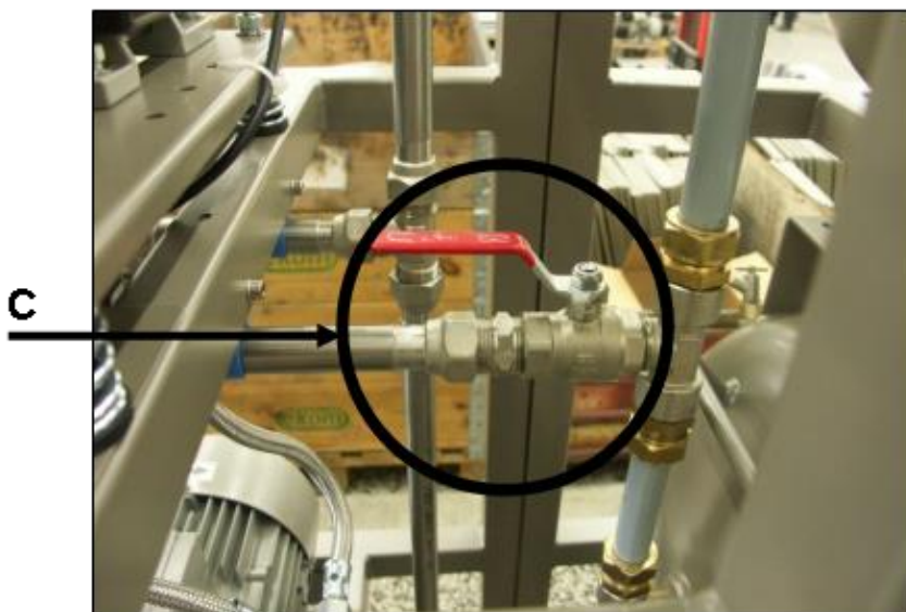
Рис. 9: Пневматические соединения
