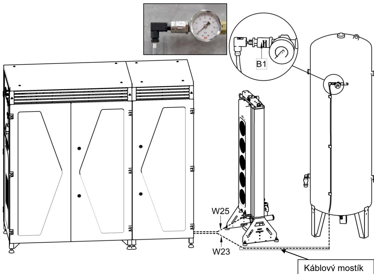
Obr. 22: Elektrická šnúra
