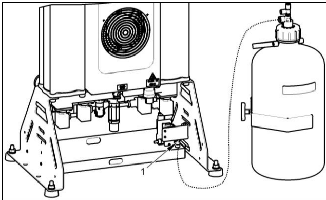
Obr. 17: Výstup kondenzátu
