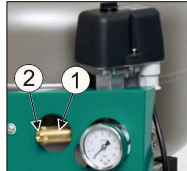
Abb. 20: Sicherheitsventil überprüfen
