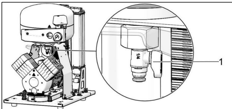
Abb. 19: Kondensatablauf
