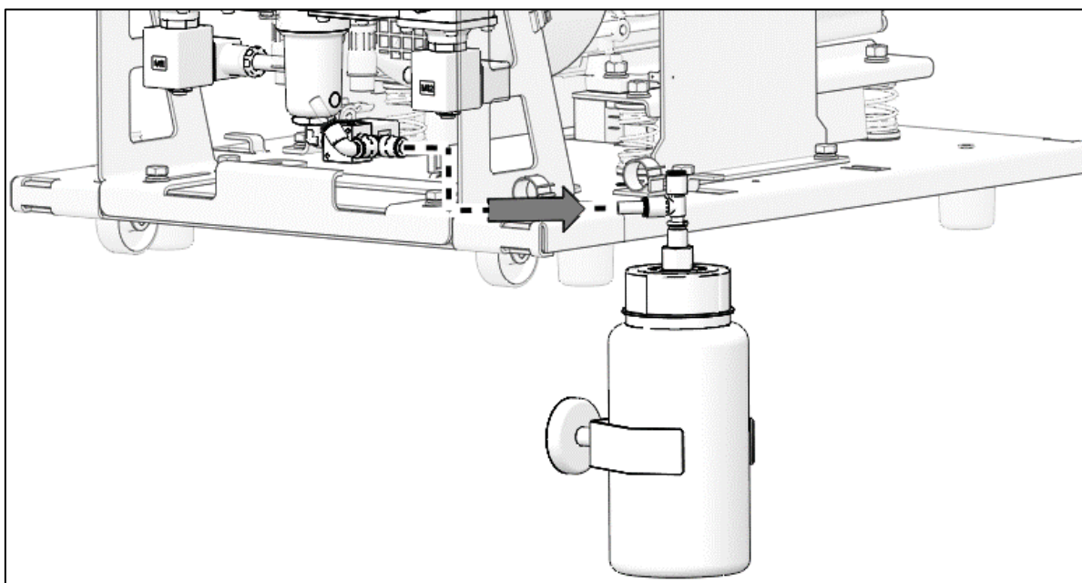
Obr. 8: Pripojenie nádoby na kondenzát
