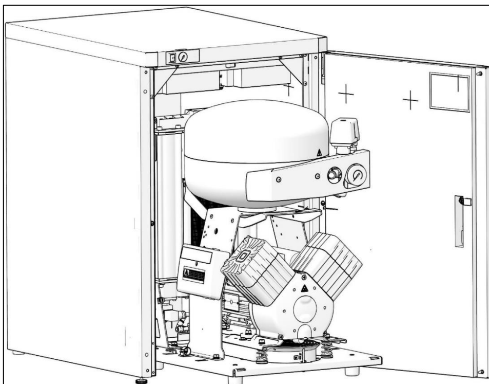
Rys. 13: Umiejscowienie sprężarki umożliwiającej wykonanie połączeń elektrycznych
