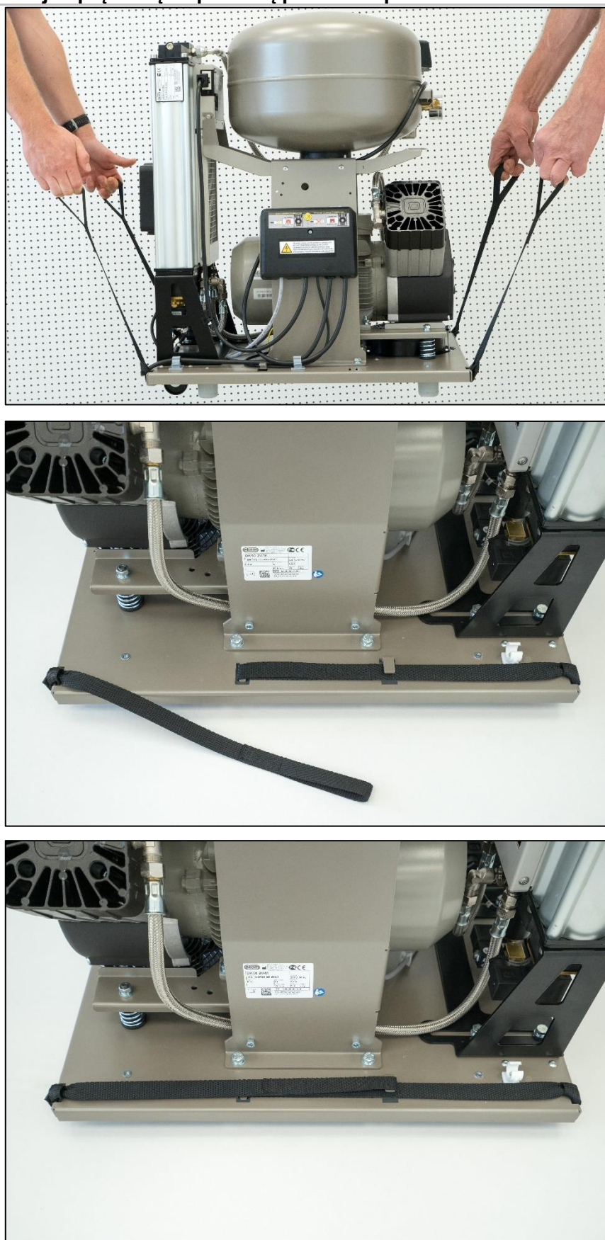
Rys. 4: Manipulacja sprężarką za pomocą pasów do przenoszenia
